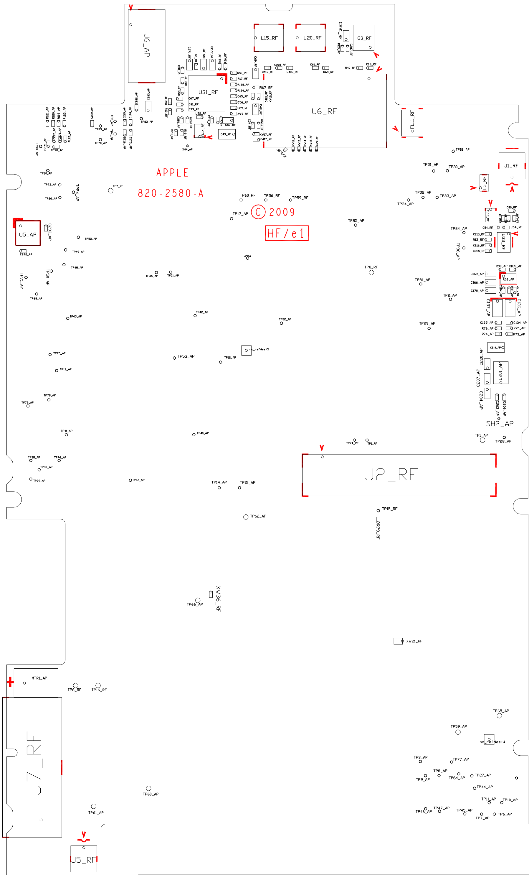
N88 MLB PVT PCBA 零件位置圖 (820-2580-A) Bot side
