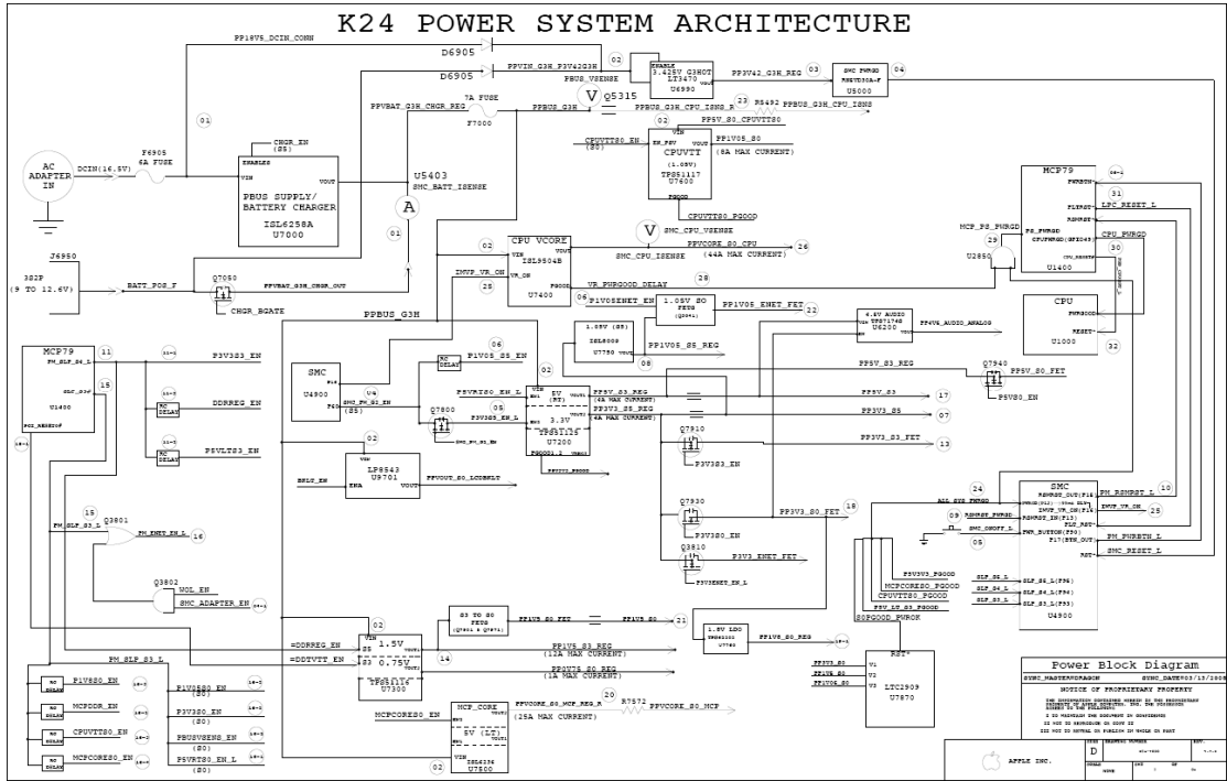
(K24 供电系统架构图)
